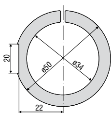
MA 2405-34: 다음 센서에 적용 IFS2405-3 IFD2415-3
