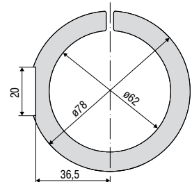
MA 2405-62: 다음 센서에 적용 IFS2405-28 / -30
