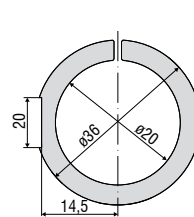
MA 2406-20: 다음 센서에 적용 IFS2406-2,5 IFS2406/90-2,5
