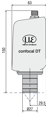
치수: mm, 실제 크기과 상이
