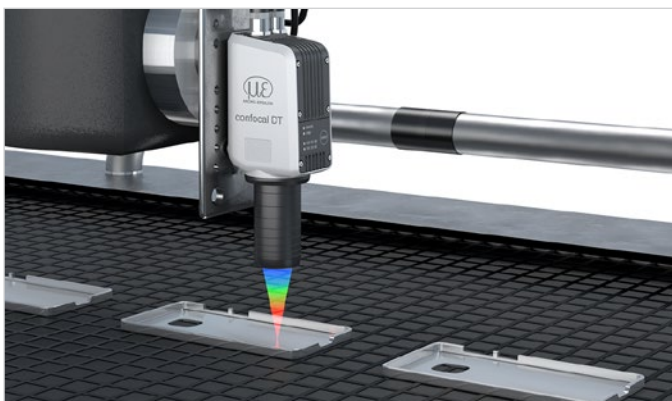
스마트폰 하우징의 인라인 측정
